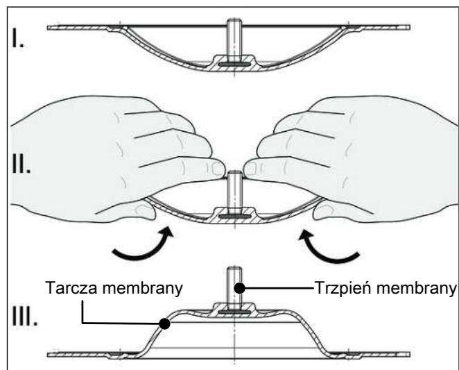
Rys. 3: Odwiniecie tarczy membrany
