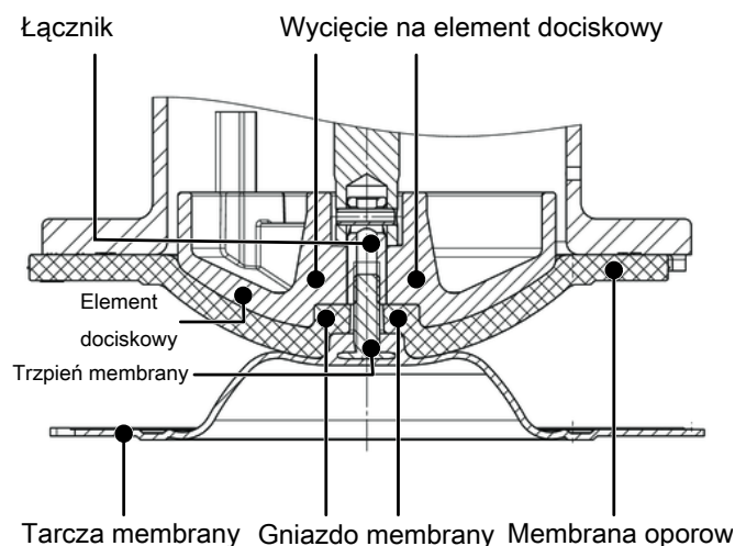
Rys. 4: Wkręcenie tarczy membrany
