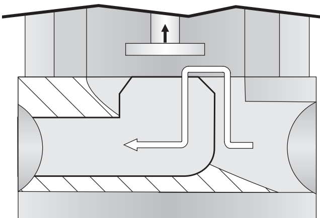
Abb. 2: Ventil OFFEN
