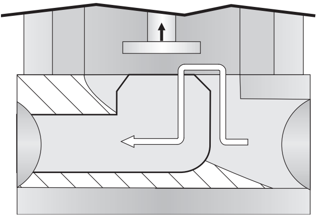
Fig. 2: Vanne OUVERTE
