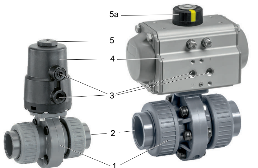
Привод GEMÜ 9415
