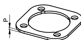
Distanzstück (DIS)
