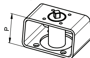
Montagesatz (MSC)
