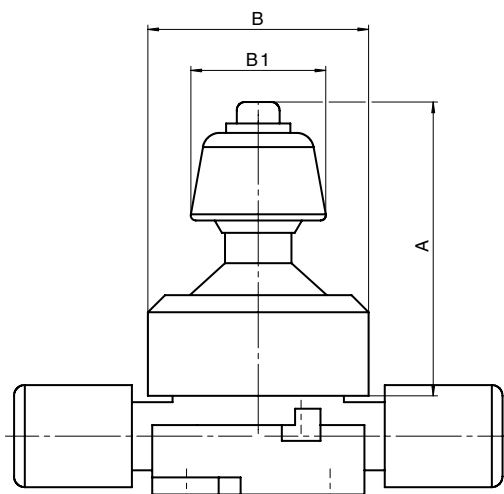
Medidas del actuador GEMÜ C67 HPW [mm/inch]
