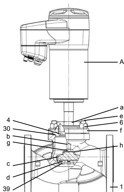
Fig. 6: Pièces détachées
