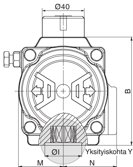
Tyyppi 0015U-1200U
