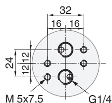
Yksityiskohta X ADA/ASR 2100U-4000U
