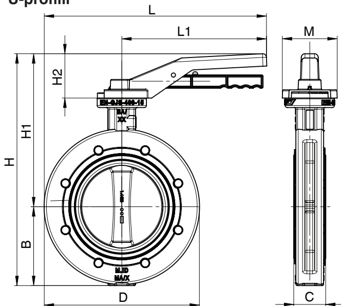
U-profiili
