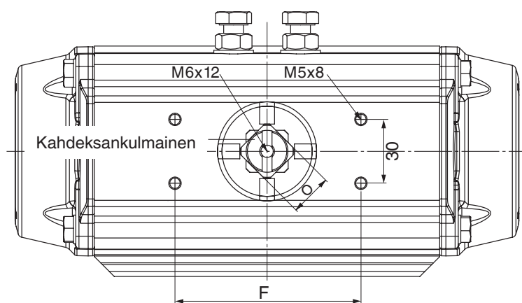
Tyyppi 0015U-1200U
