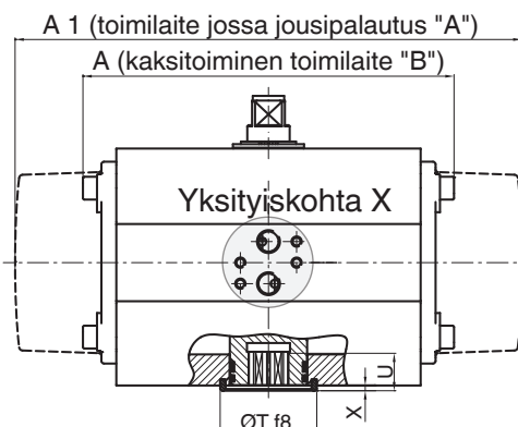
Yksityiskohta X ADA/ASR 2100U-4000U
