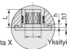
Tyyppi 5000U
