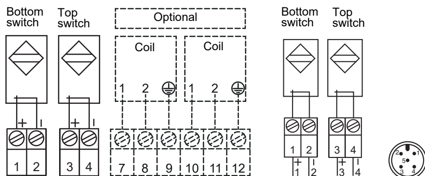
M12 Anschlussvariante
