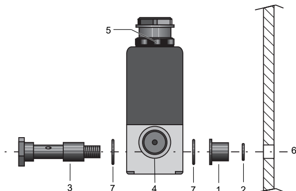
илл. 1: Монтаж GEMÜ 0324
