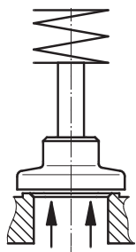
Actionneurs 0, 1, 2 flux sous le clapet*
