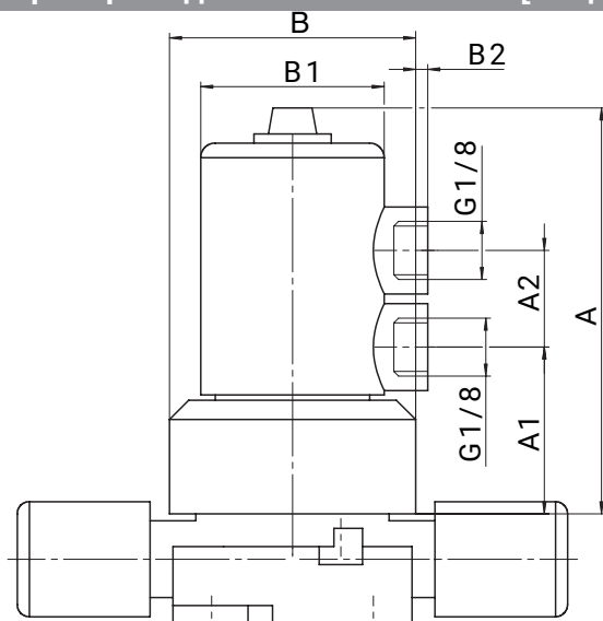
Размеры привода GEMÜ C60 HPW [мм/дюйм]
