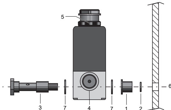
Rys. 1: Montaż GEMÜ 0324
