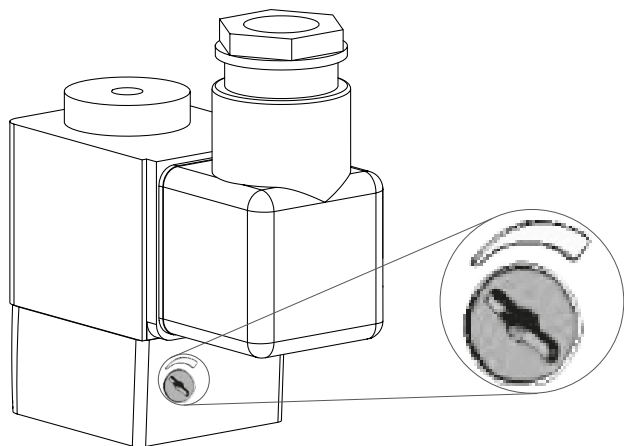
Rys. 4: Ręczne sterowanie awaryjne
