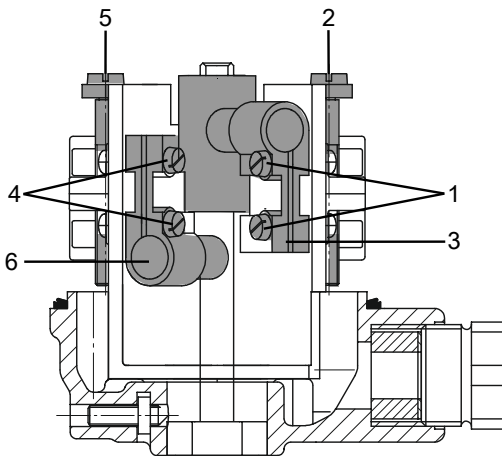
Bild1: Schaltposition einstellen
