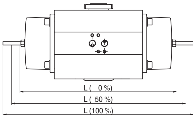
Pogon s mogućnosti krajnjeg položaja ovisnog o okretnom kutu (100 %)
