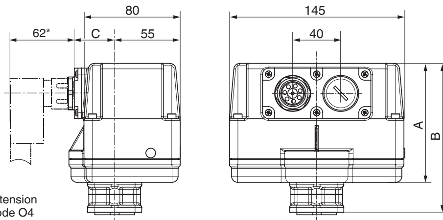
Type d'actionneur 1015
