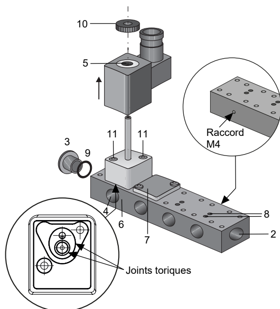
Fig. 1: Montage GEMÜ 0326
