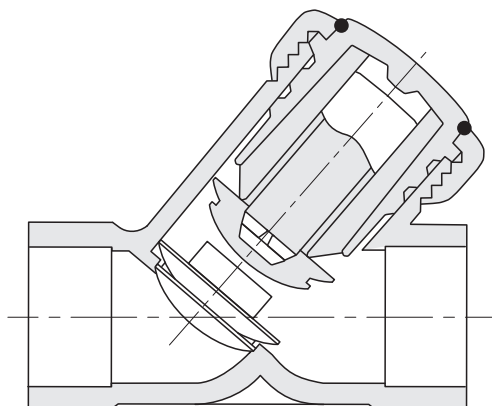
Schnittbild
