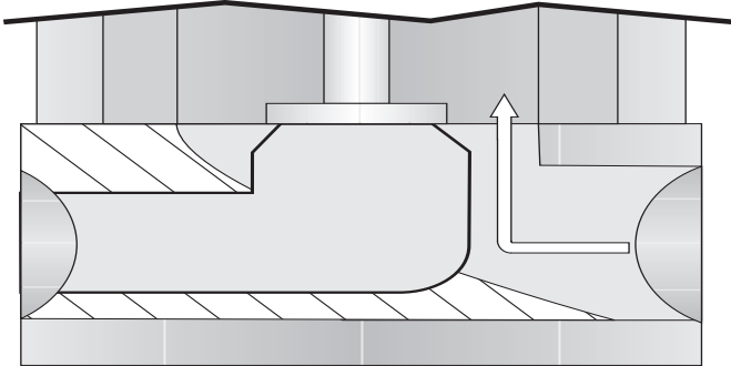
Abb. 1: Ventil GESCHLOSSEN
