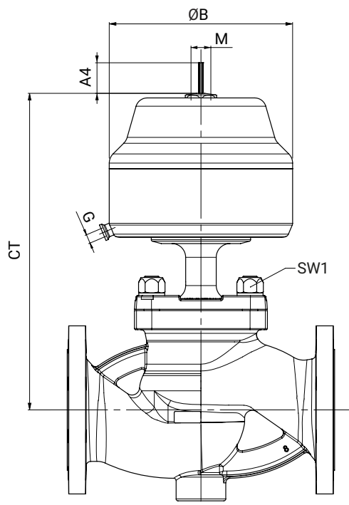
Taille d'actionneur 6
