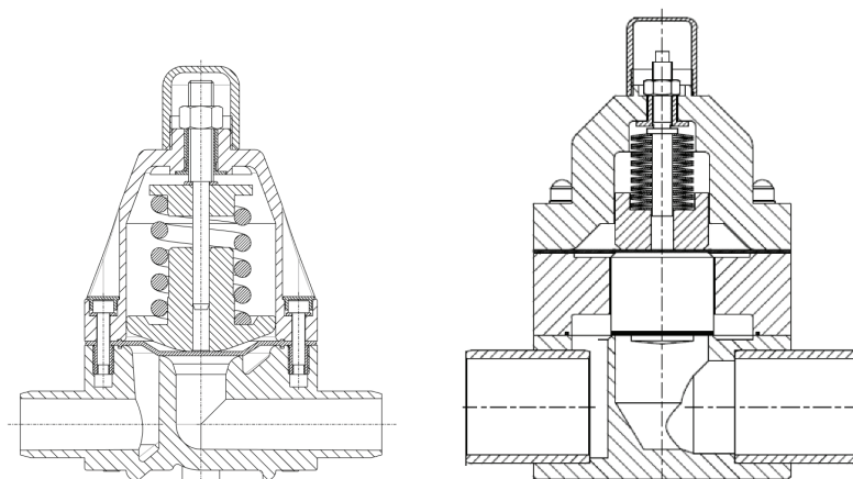
DN 10-50
