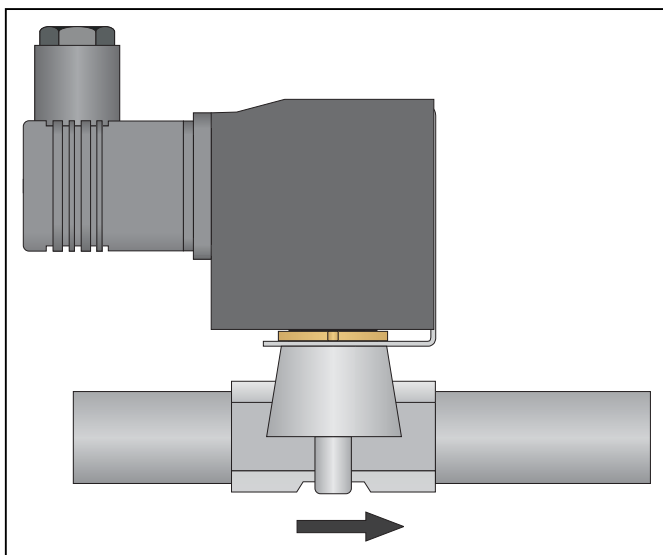
Установка электромагнитного клапана
