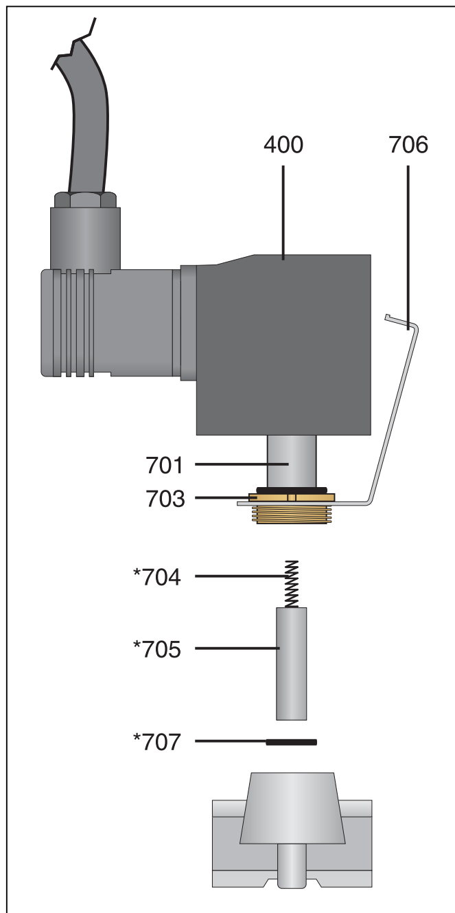
Замена якоря электромагнита
