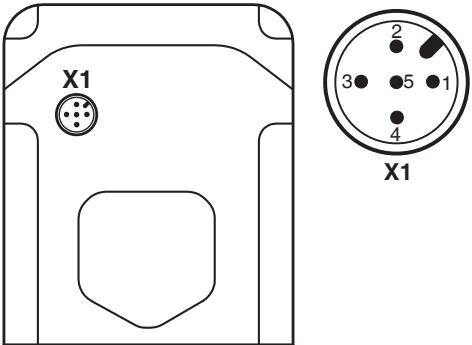
Elektrische Anschlüsse
