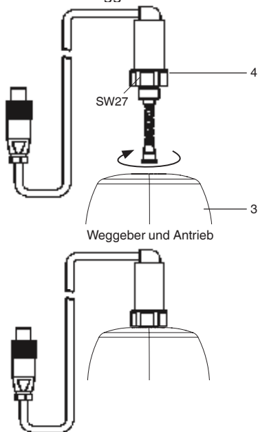
Weggeber auf Antrieb montiert
