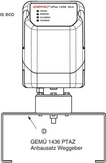
Direkter Anbau an Schwenkantrieb
