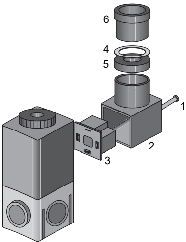
Fig. 3: Connexion électrique - Connecteur femelle
