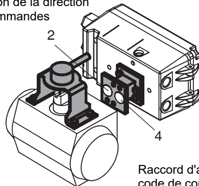
Raccord d'air de pilotage code de commande ...VT
