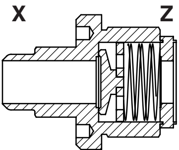
Clapet anti-retour, raccord flare + filetage UN sens du passage de X à Z Type Code CVFU
