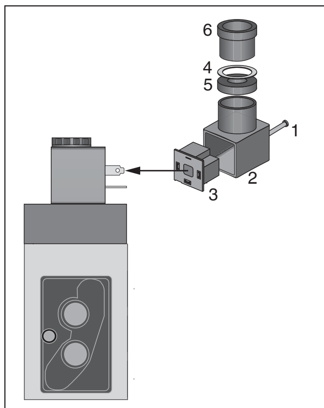
Connexion électrique
