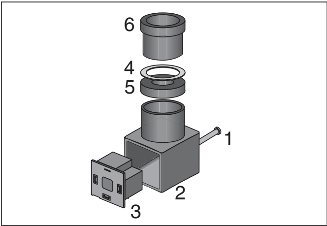
Connecteur femelle
