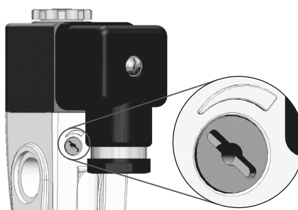
Abb. 5: Handnotbetätigung
