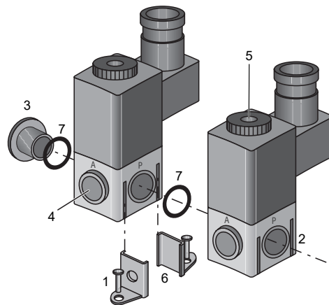
Abb. 2: Batteriemontage GEMÜ 0322
