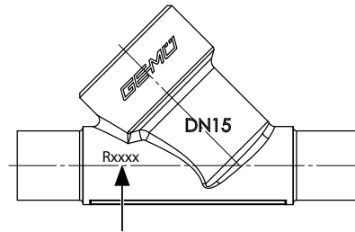
Identificación del cuerpo de la válvula Cuerpo paso recto
