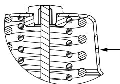
Orificio de venteo estándar
